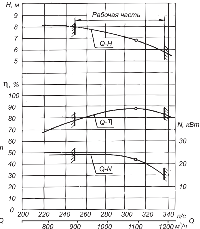
Характеристика насоса О-35-1100Г
