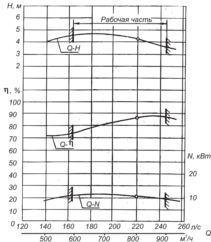
Характеристика насоса О-35-800Г
