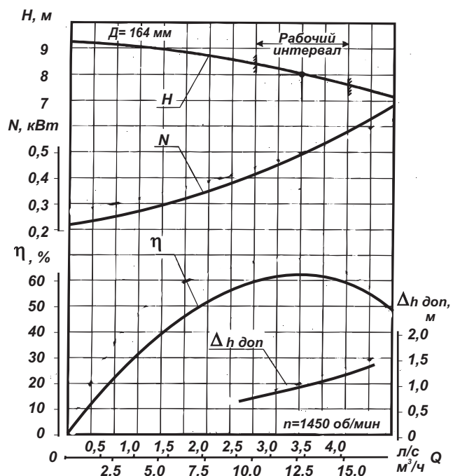
Характеристика насоса НД 80-50-160/4
