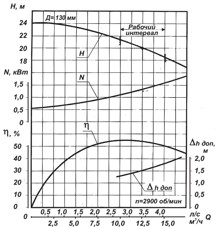
Характеристика насоса НД 80-50-125
