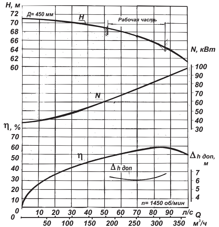
Характеристика насоса КТС 250-67
