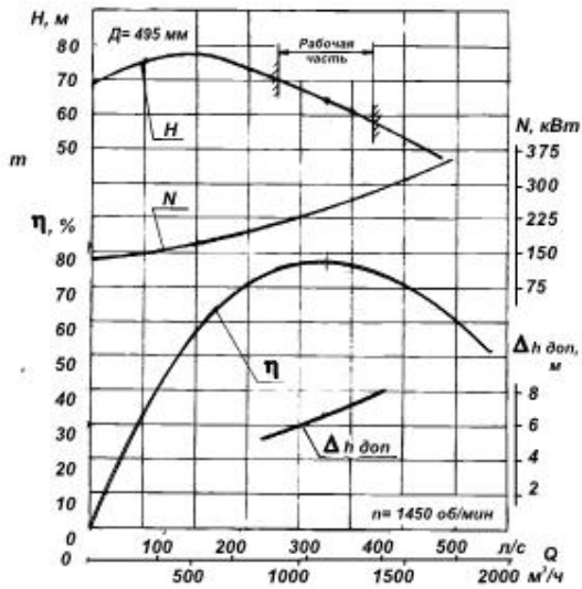
Характеристика насоса ДФ 1100-63
