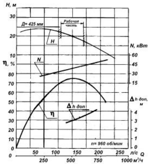
Характеристика насоса ДФ 700-23
