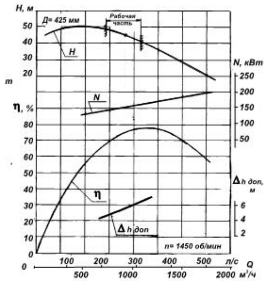
Характеристика насоса ДФ 1100-63
