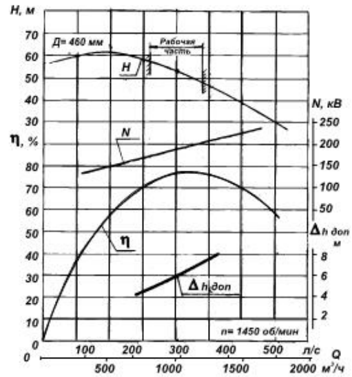
Характеристика насоса ДФ 1000-53
