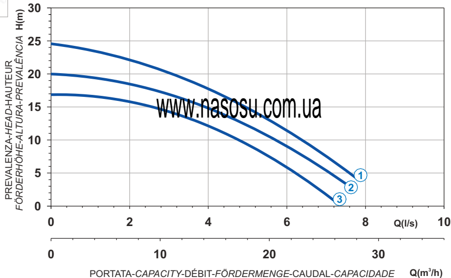
Curva caratteristica - Performance curve - Courbe caractéristique Kennlinie - Curva caracteristica - Curva caracteristica
